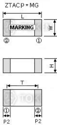
MHz (ZTACP*MG) Dimensions
