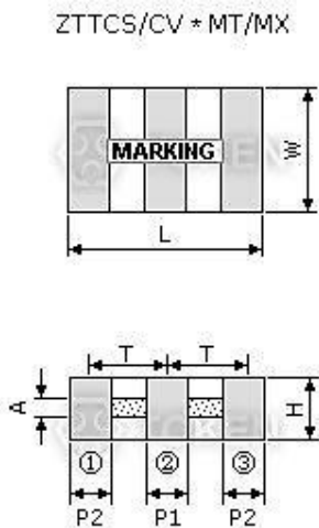
MHz (ZTCS/CV*MT/MX) Dimensions
