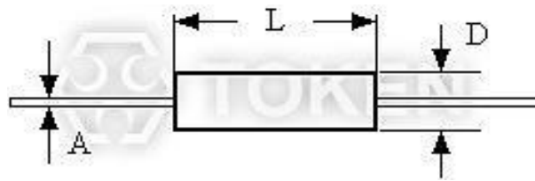
(UAR) Dimensions
