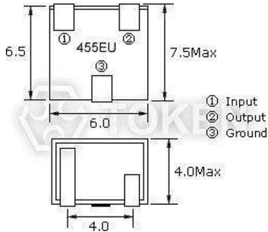
(LTC 455EU) Dimensions
